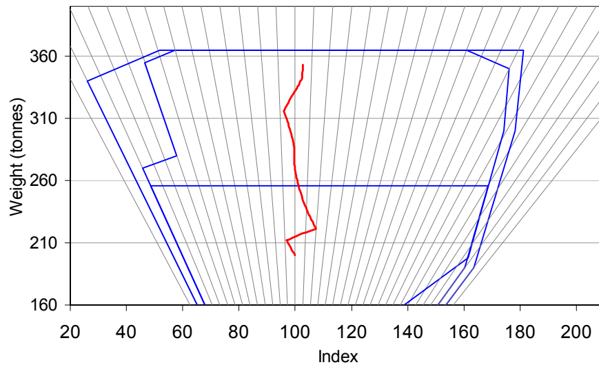
A340-600
