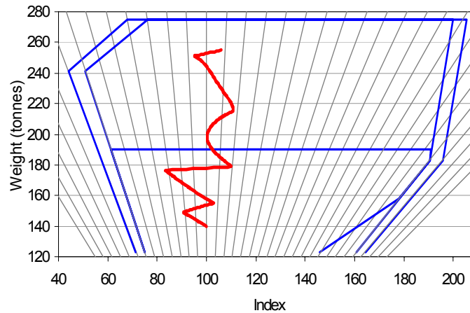
A340-200/-300 (1 ACT)
